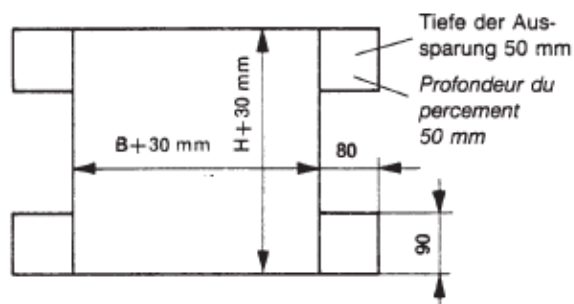
Aussparungsplan
