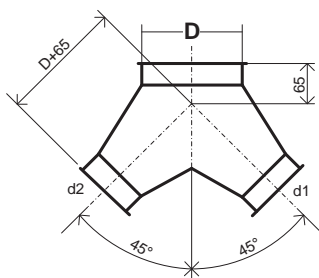
Hosenrohr 45° Culotte 45°
